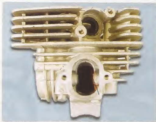
Culata 4T de refrigeración directa
